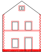
12001 - ET6 1 Stück Hauptwand straßenseitig
